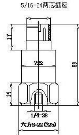
外形尺寸
